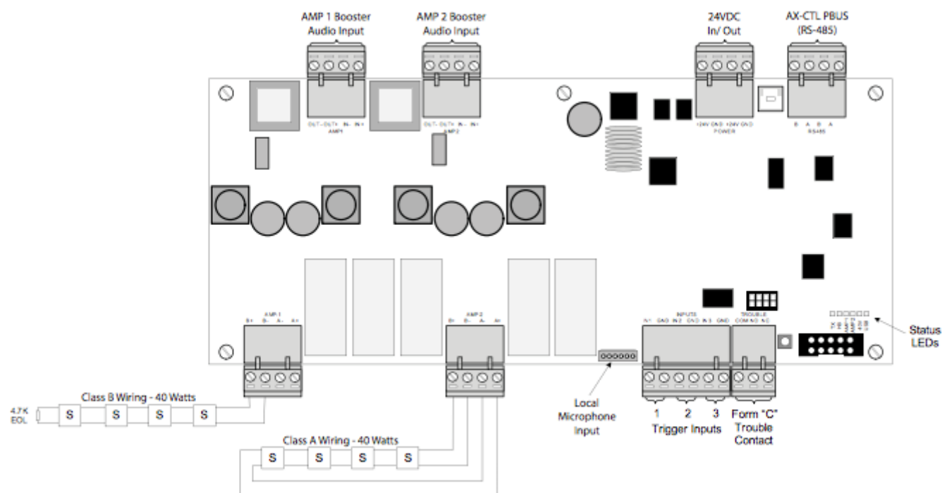
AV-AMP-80 Wiring
