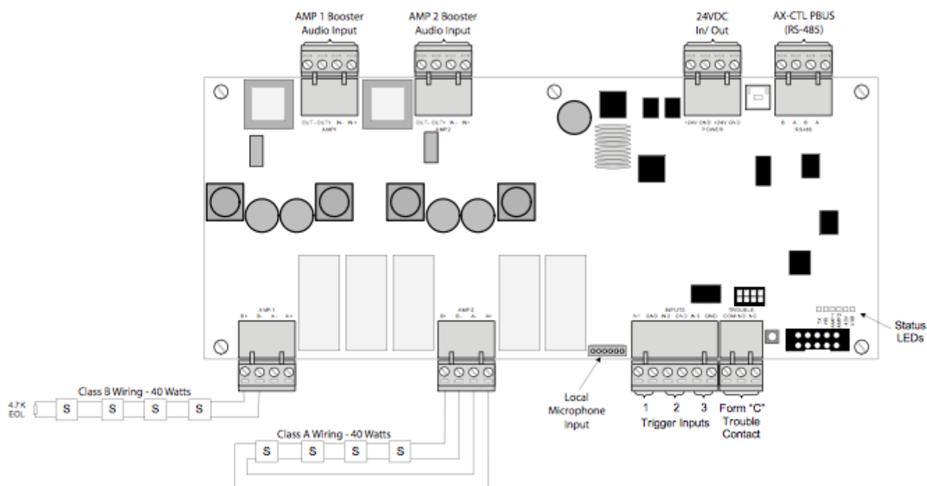
AV-AMP-80 Wiring
